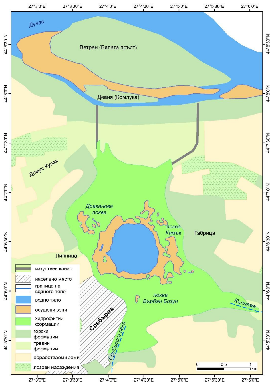
Фиг. 5. Пространствен модел на съвременната ландшафтна структура на влажната система „Сребърна“. Земното покритие в прилежащите територии е представено по данни от CORINE Land Cover (CLC) 2018 (изготвил: Юлиан Тотев).
