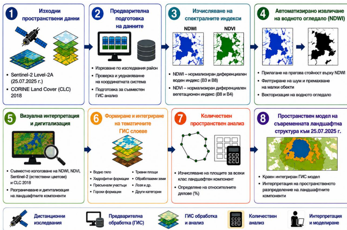
Фиг. 3. Методическа схема на пространственото моделиране на съвременната ландшафтна структура на влажната система „Сребърна“
