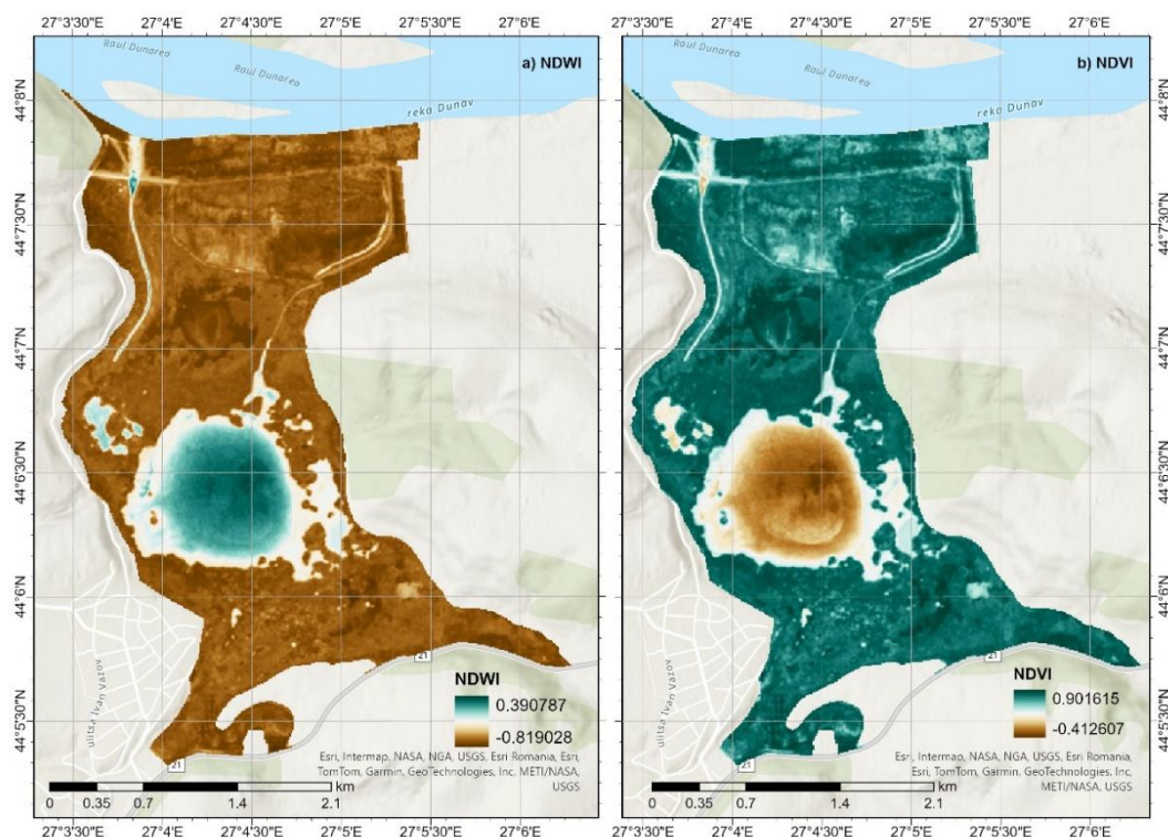
Фиг. 4. Пространствено разпределение на: а) нормализирания диференциален воден индекс (NDWI) и б) нормализирания диференциален вегетационен индекс (NDVI) в района на влажната система „Сребърна“ по данни от Sentinel-2 L2A от 25 юли 2025 г.
